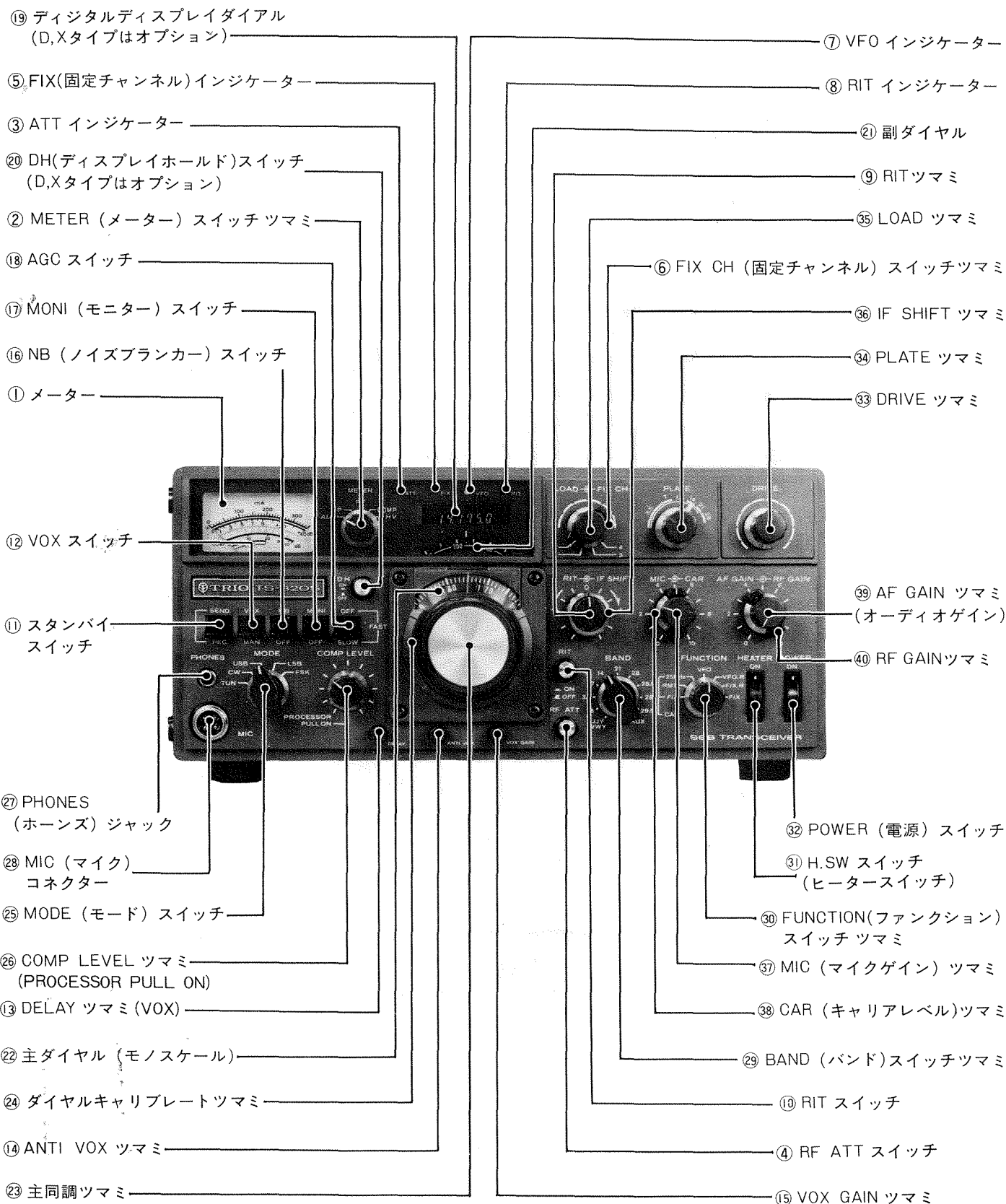
前面パネル
